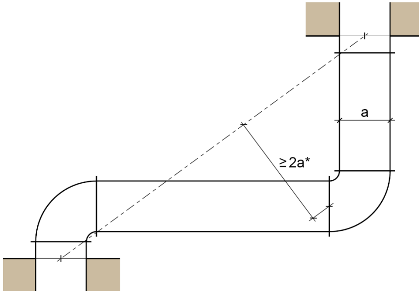
Bild 5.1: Begrenzung der Krafteinleitung mit Leitungsverziehung
